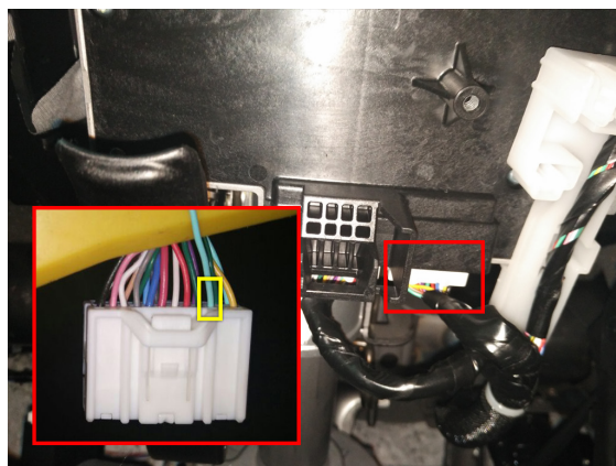
Рис.3 Подключение зажигания
