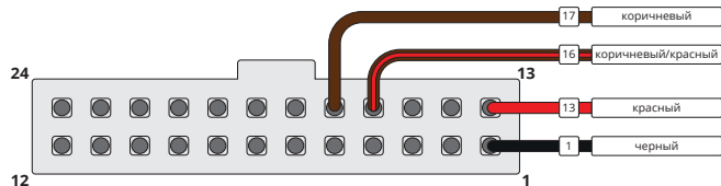
Рис. 2. Нумерация контактов в разъеме, вид со стороны проводов
