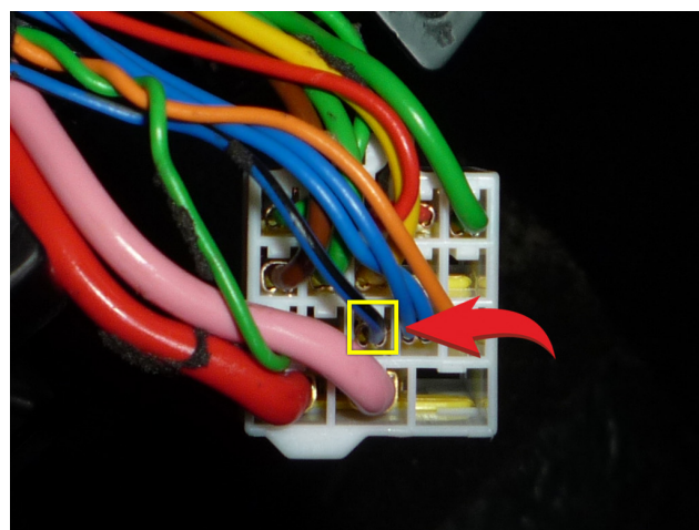
Рис.3 Шина данных (синий/черный)
