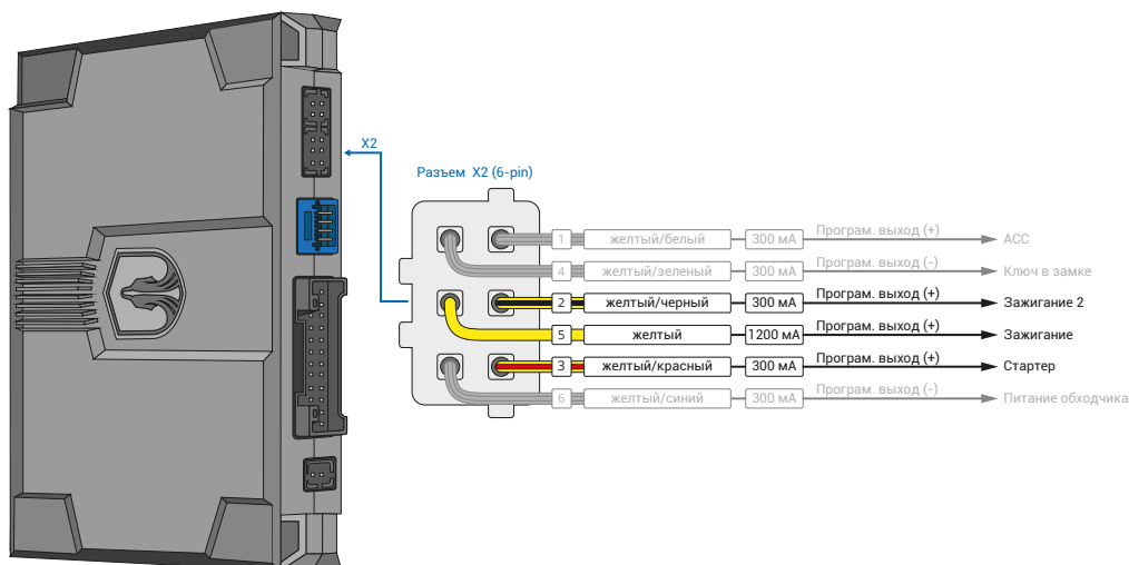
Рис.4 Подключение выходов автозапуска
