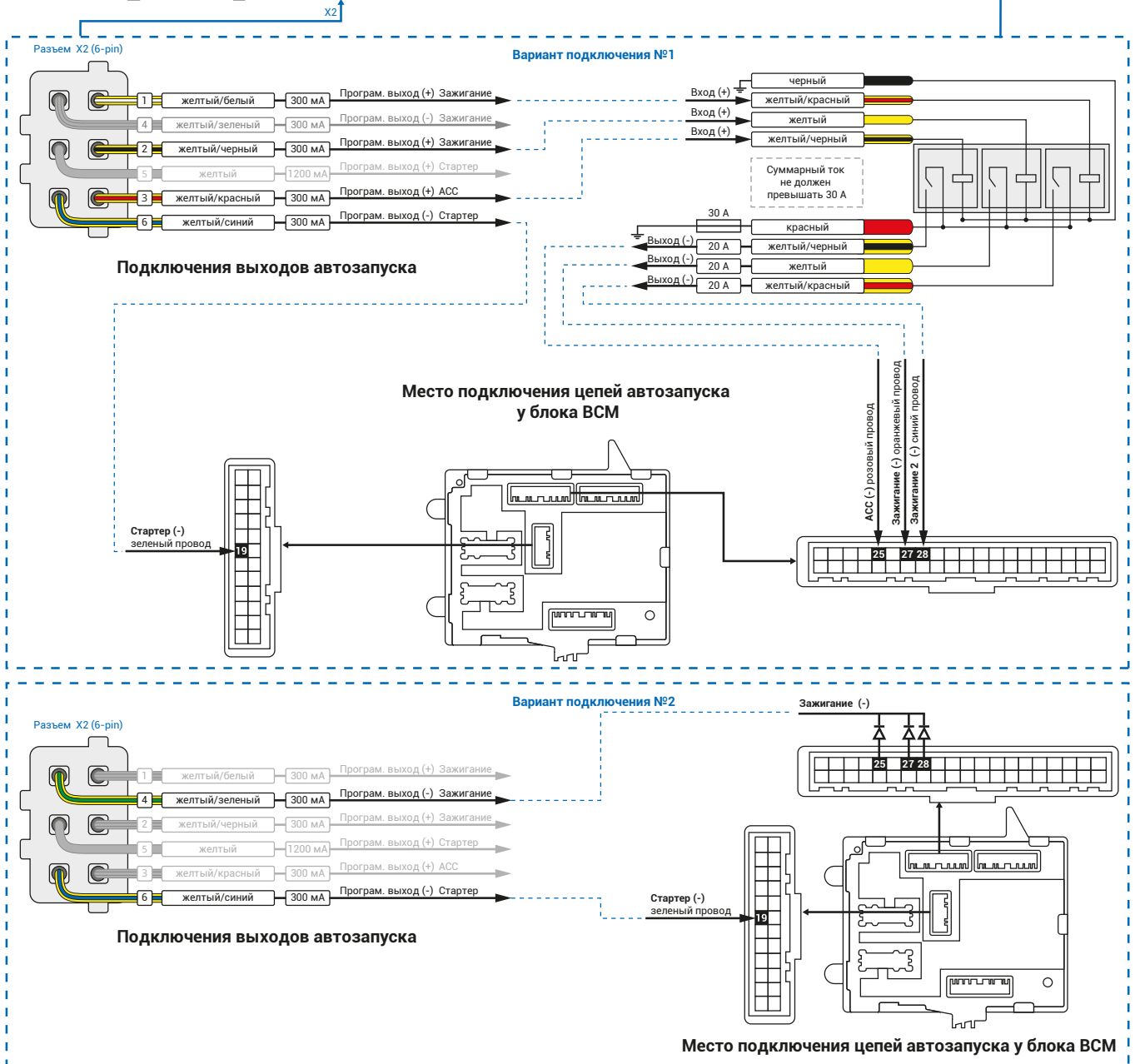
Рис.4 Схема подключения автозапуска
