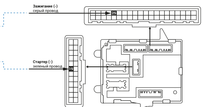
Рис.4 Схема подключения автозапуска
